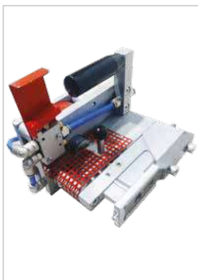
Poinçonneuse 80 - 67 - 22+40
