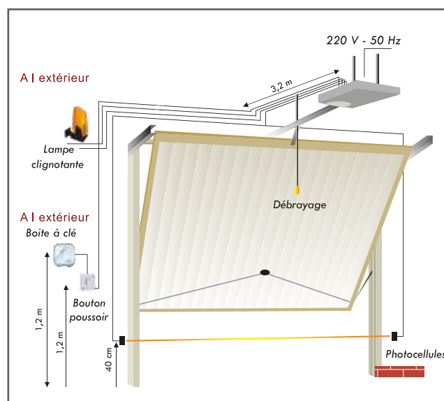
Porte Basculante
