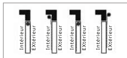
Positionnement des enroulements
