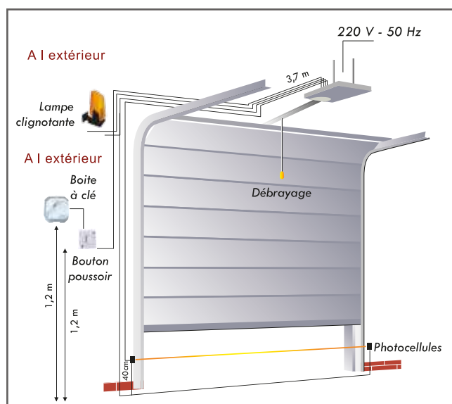
Porte Sectionnelle
